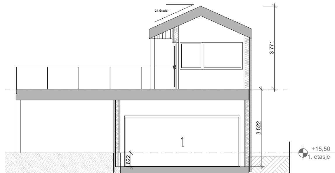
1:100 Snitt B
