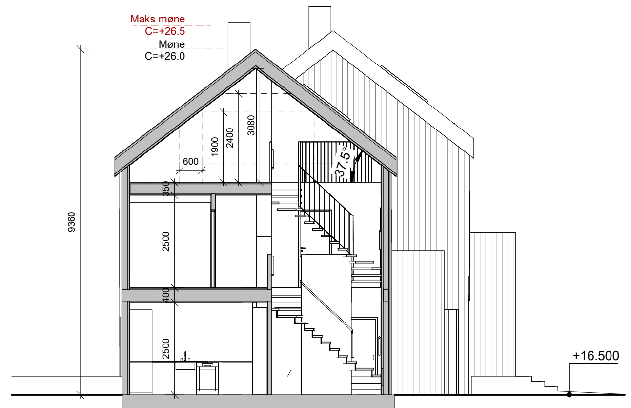
Tverrsnitt nr. 46
